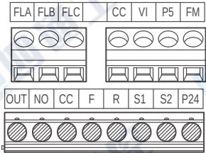
控制电路端子
